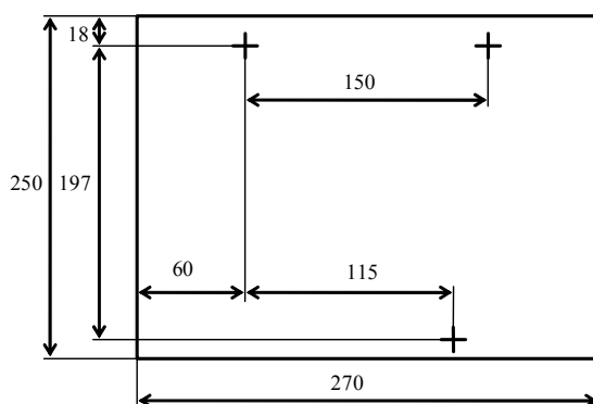
Рисунок 2. Разметка для крепления ППКОПП.
