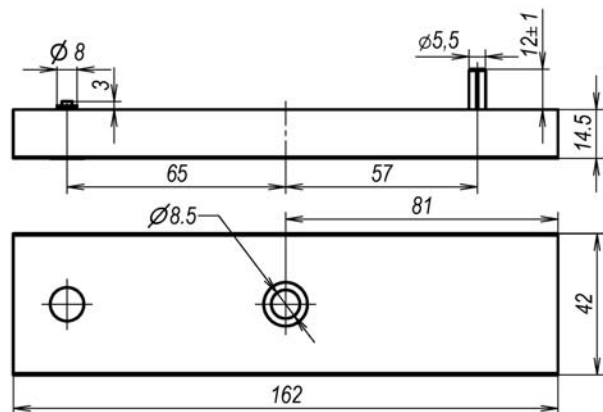
Рис. 6 Якорная часть
