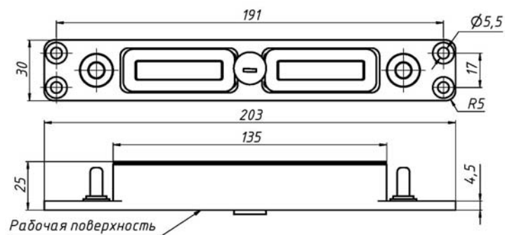
Рис.5 Корпусная часть.
