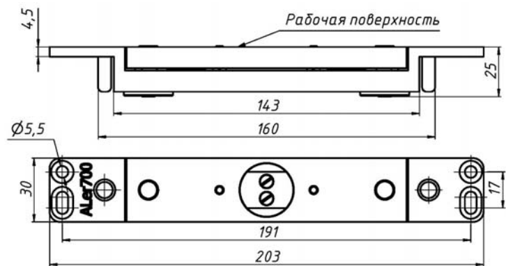
Рис.4 Якорная часть.
