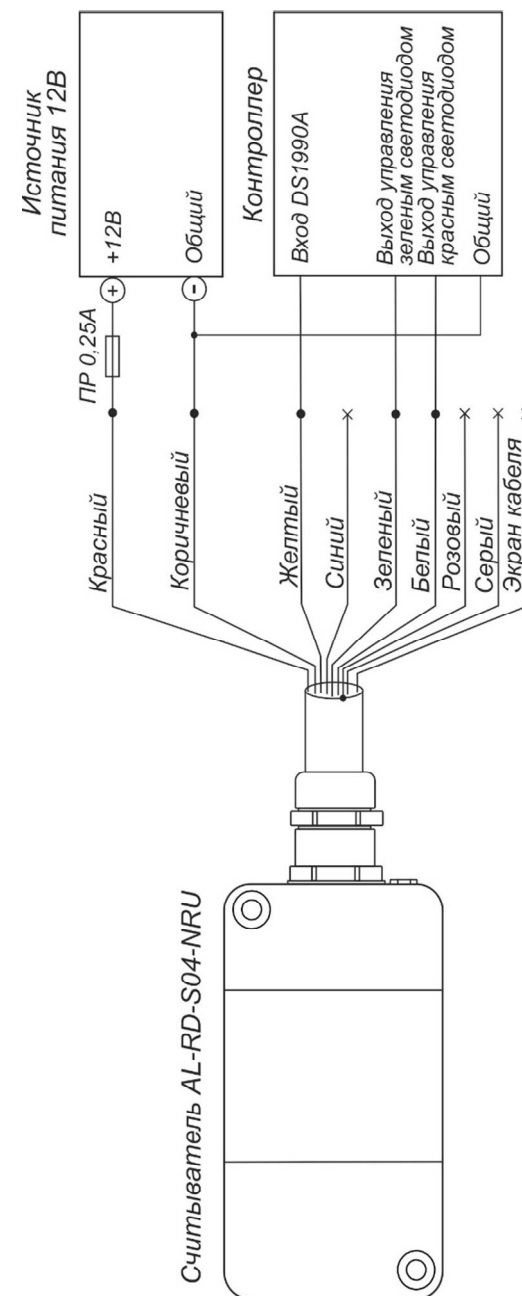
Рис.1. Схема подключения считывателя в режиме DS1990A.
