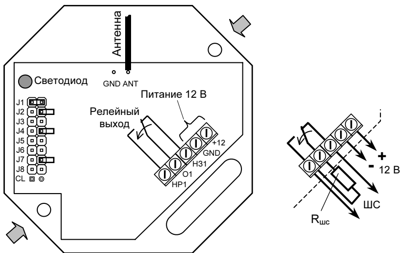
Рисунок 2. Монтажная схема приемника и пример монтажа шлейфа
