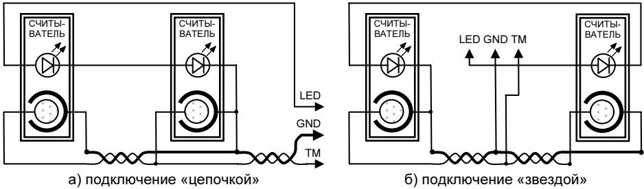
Рисунок 3. Подключение двух считывателей
