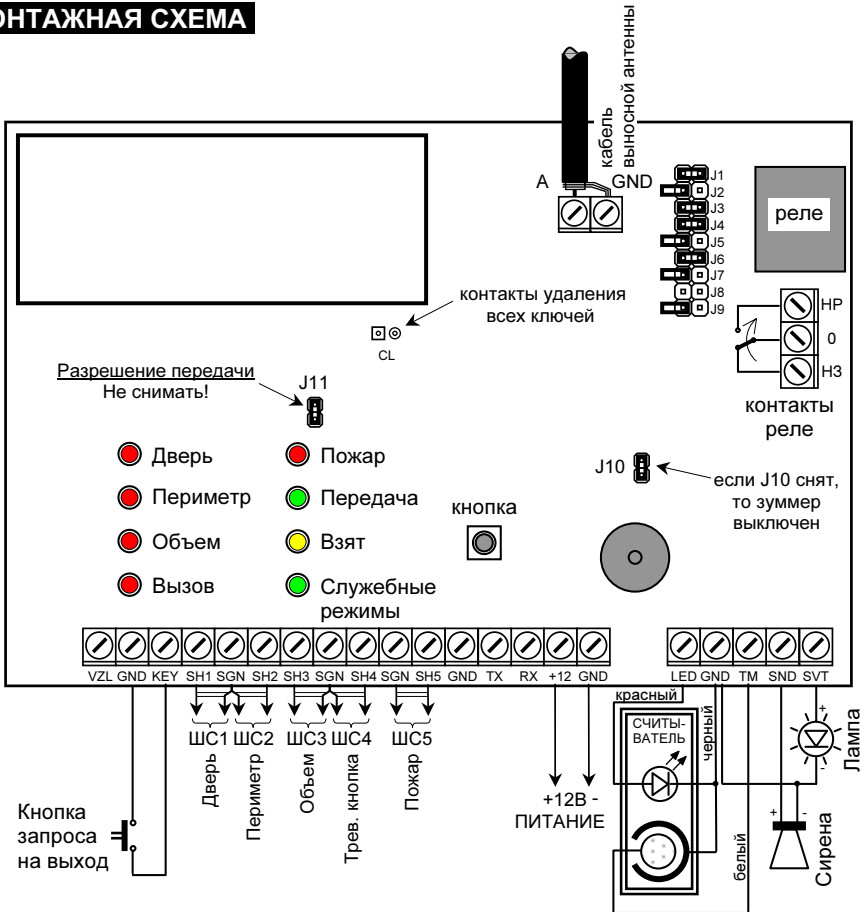
Рисунок 5. Монтажная схема передатчика
