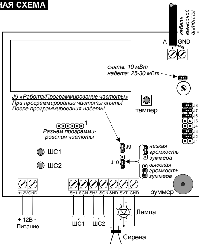
Рис. 5. Монтажная схема передатчика
