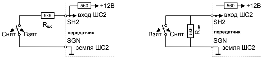
Рис. 4. Примеры монтажа ШС2 в качестве входа постановки/снятия с охраны
