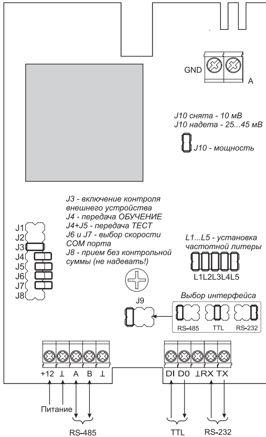
Рис. 2. Монтажная схема передатчика
