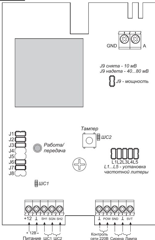
Рис. 6. Монтажная схема передатчика
