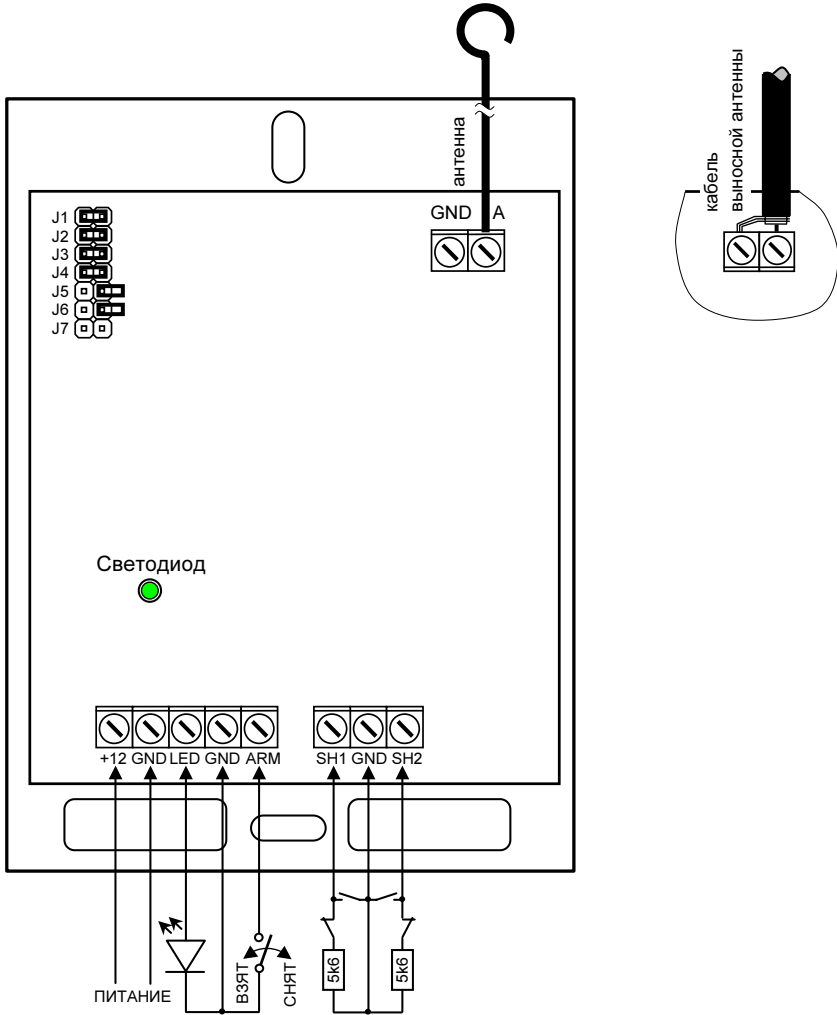
Рис. 2. Монтажная схема передатчика и подключение антенны
