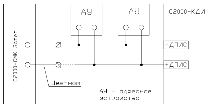
Рис. 1 Схема соединений
