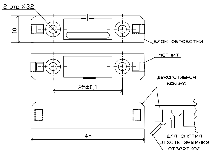
Рис. 2 Установочные размеры
