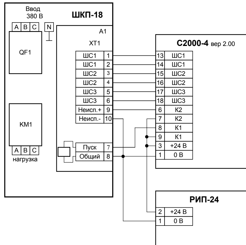
Рис. 2 Пример подключения шкафа "ШКП-18" к прибору С2000-4
