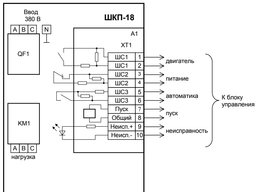
Рис 1 Схема электрическая подключения шкафа "ШКП-18" при эксплуатации
