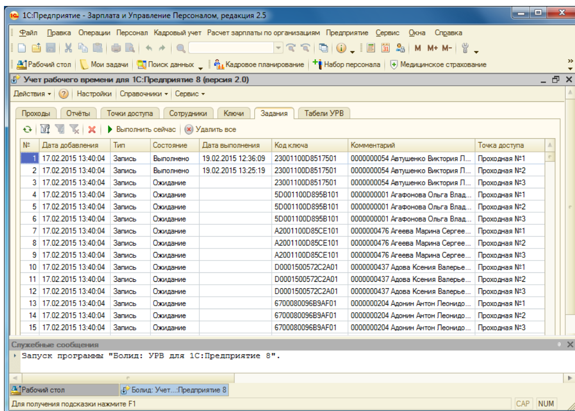
Рисунок 3.14. Страница «Задания».
