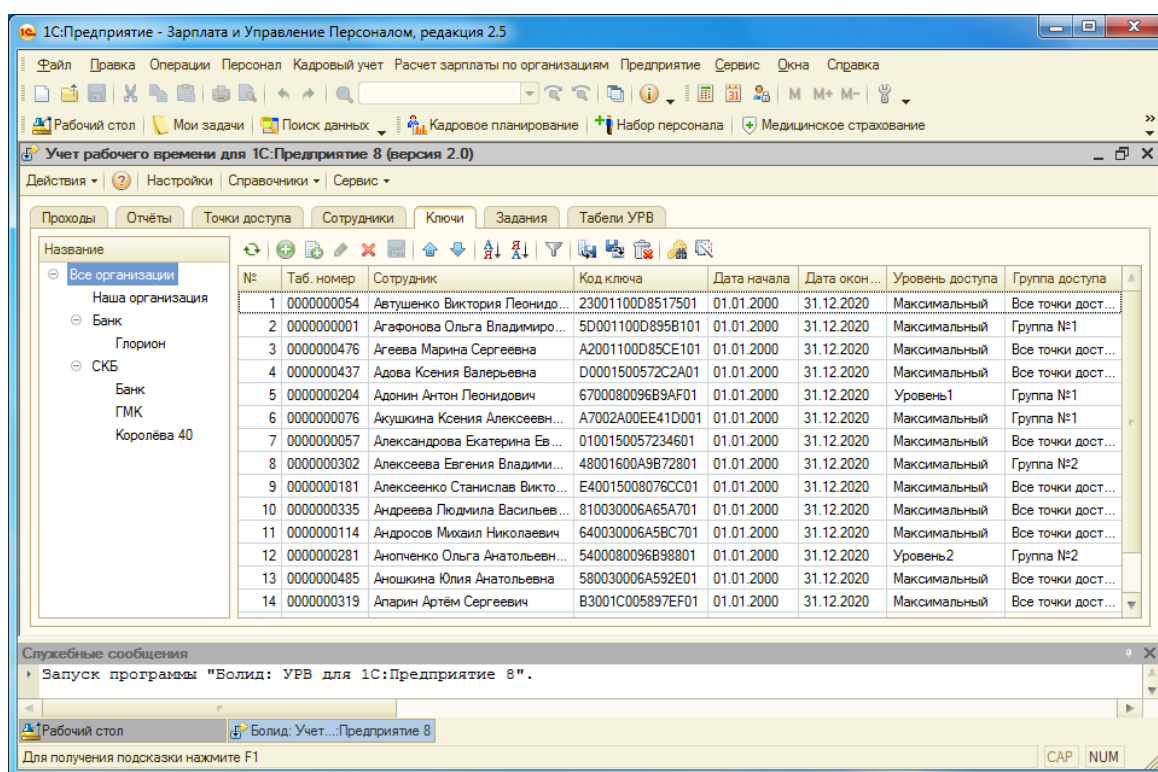
Рисунок 3.12. Страница «Ключи».
