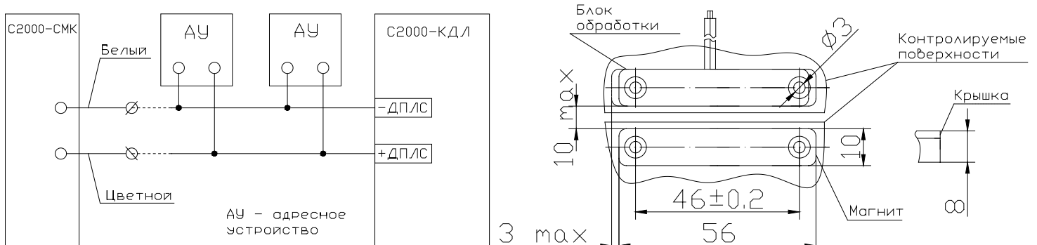
Рисунок 1 Схема соединений
