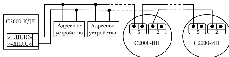
Рисунок 1. Схема соединений
