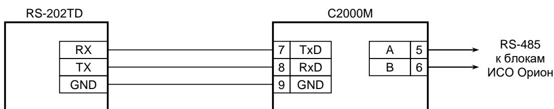
RS-202TD – радиопередатчик «Риф Стринг RS-202TD-RR»; C2000M - пульт контроля и управления «С2000М».
