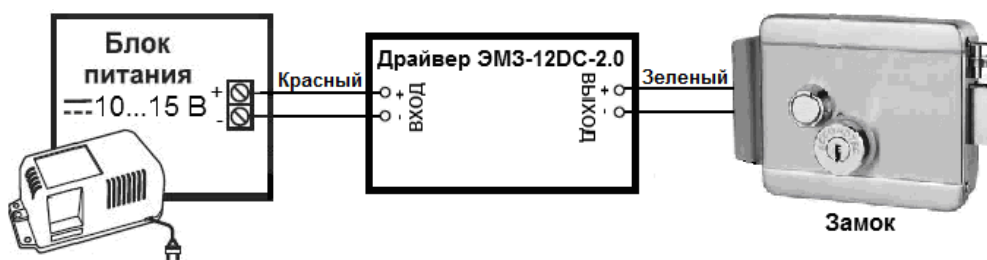
Рис.1. Вариант подключения драйвера.
