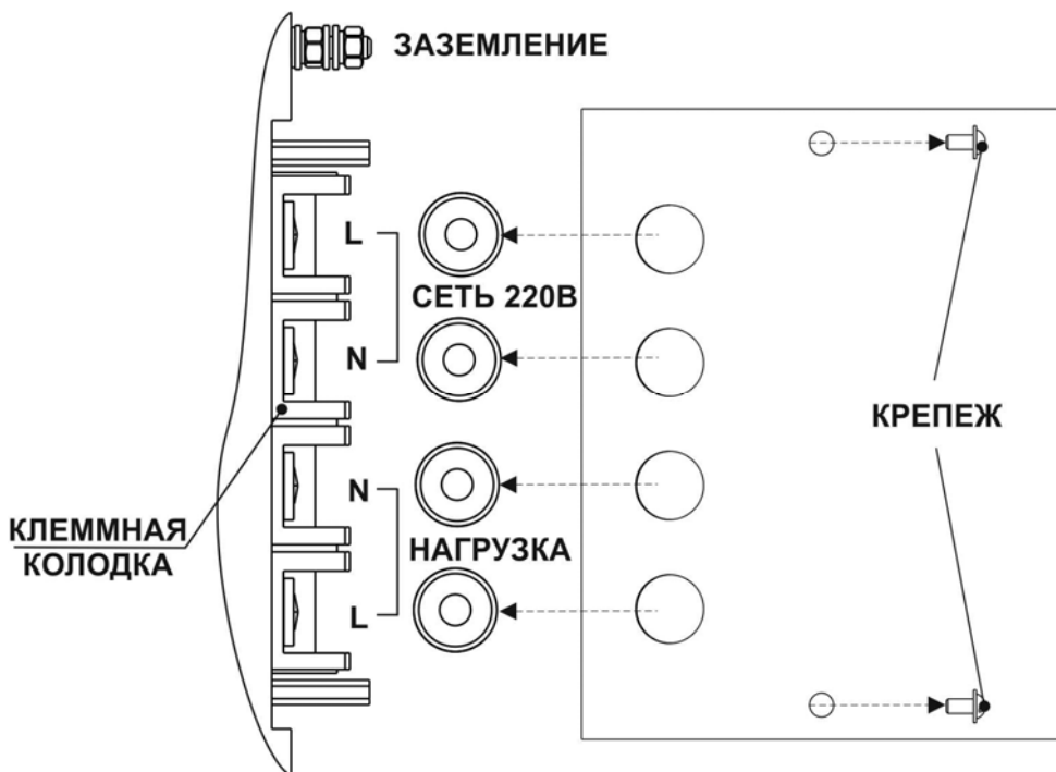
Рисунок 3 – Подключение изделия
