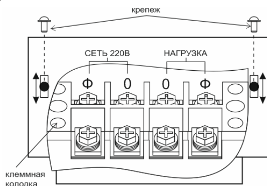
Рисунок 3 – Схема подключения к клеммной колодке
