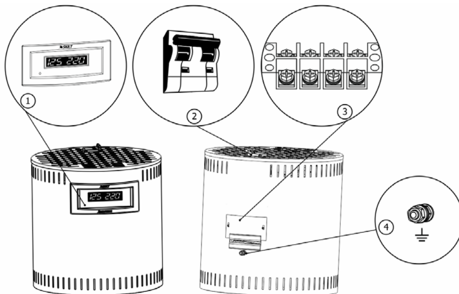
Рисунок 1 Общий вид стабилизатора и его функциональных элементов
