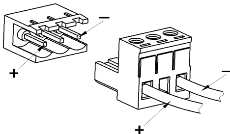
Рисунок 1. Подключение нагрузки к розетке «12 В» с помощью разъёма 2EDGK-5.0-03P.
