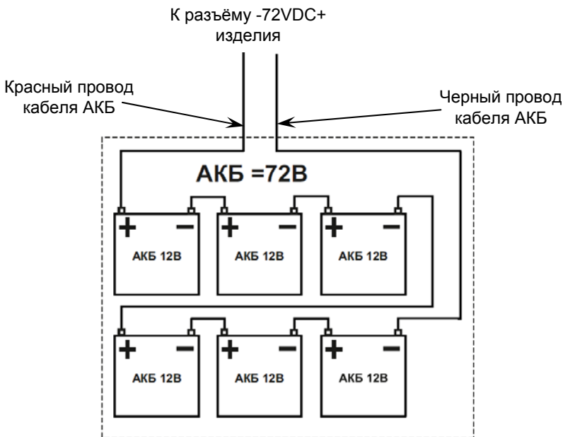
Рисунок 7 — схема монтажа аккумуляторной батареи.
