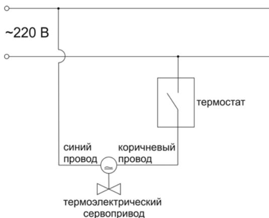
Рисунок 4 – схема подключения изделия
