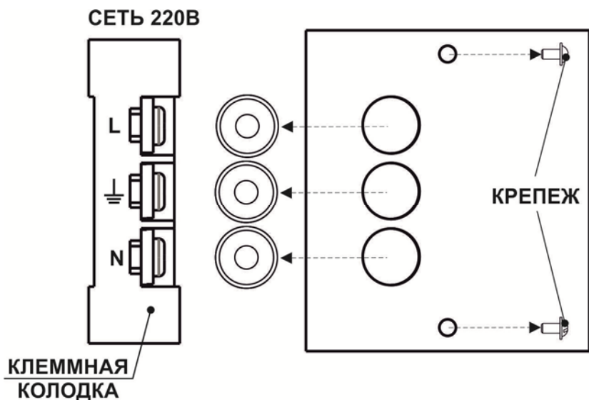
Рисунок 3 – Подключение изделия
