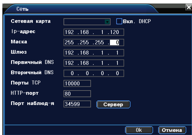
Рисунок 4.12 Сеть
