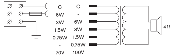
Принципиальная схема
