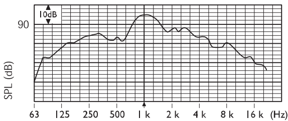
Частотная характеристика
