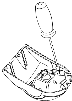
Рис 9 Замена линзы
