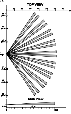
Рис 8 Диаграмма направленности линзы, обеспечивающей проход для животных
