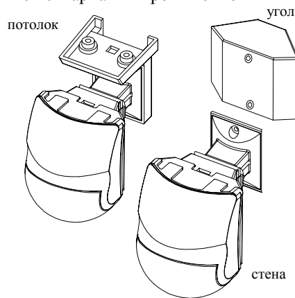
Рис 10 Варианты кронштейнов
