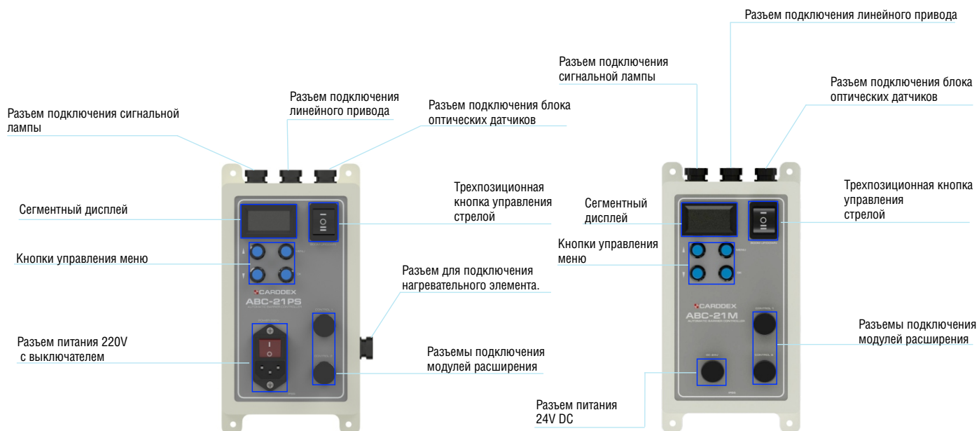
Рисунок 5. Внешний вид блоков управления «ABC-21PS» (справа) и «ABC-21M» (слева)
