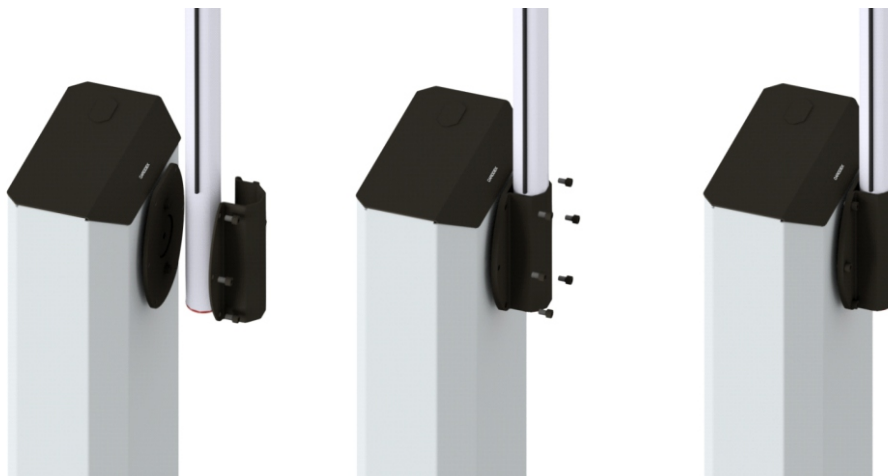
Рисунок 18 – Установка стрелы на шлагбаум
