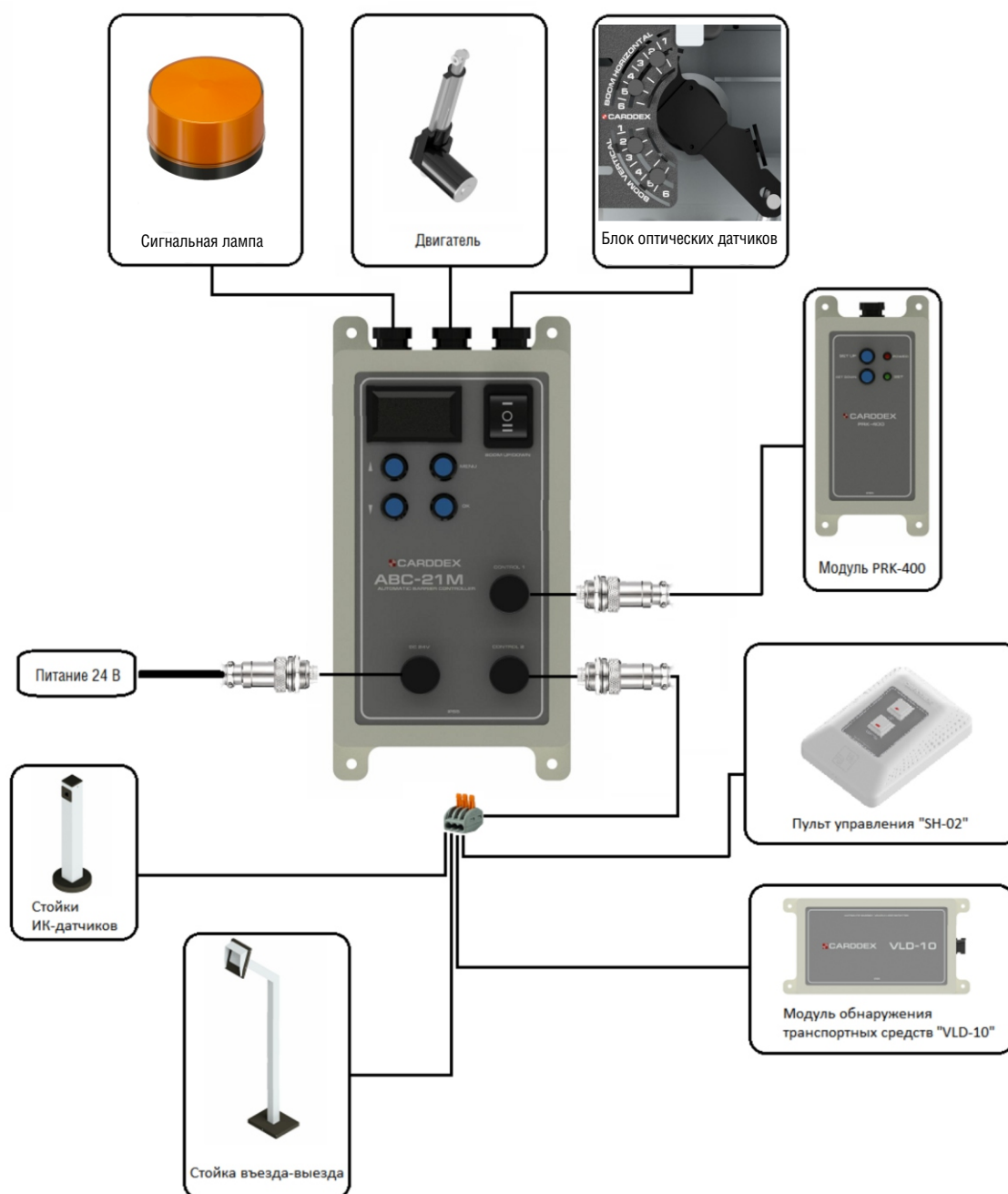
Рисунок 19 – Схема подключений устройств к шлагбауму «RBA-100»
