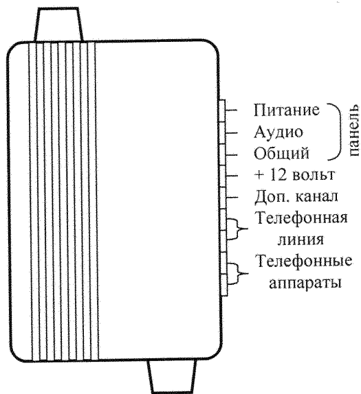
Рис. 2. Подключение МА.
