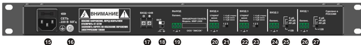
Рис. 2. Задняя панель МП. 15 – соединитель и предохранитель питания ~220В, 16 – клемма защитного заземления, 17 – клеммная колодка питания =24В, 18 – выключатель заземления, 19 –соединитель выхода, 21, 23, 25, 27 – микропереключатели уровня 4, 3, 2, 1 входа, 20, 22,24, 26 –соединители 4, 3, 2, 1 входа.
