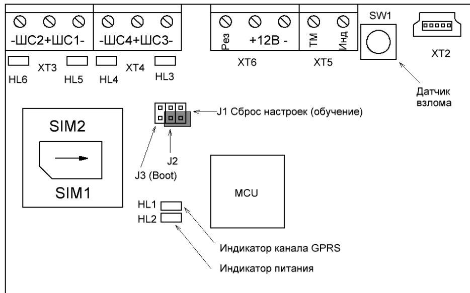
Рисунок 3.2 - Плата версии 0.2. Взаимное замыкание перемычек
