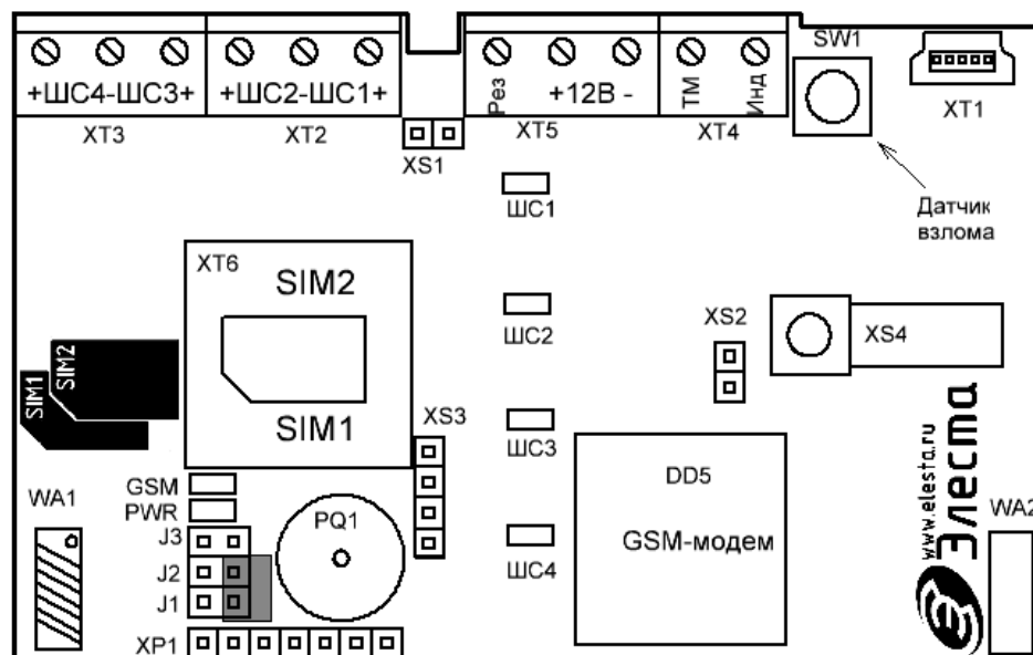
Рисунок 3.3 - Плата версии 0.6 и 0.7. Взаимное замыкание перемычек
