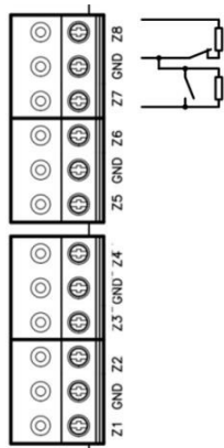
Рис. 15. Подключение шлейфов блокировки и свободного прохода
