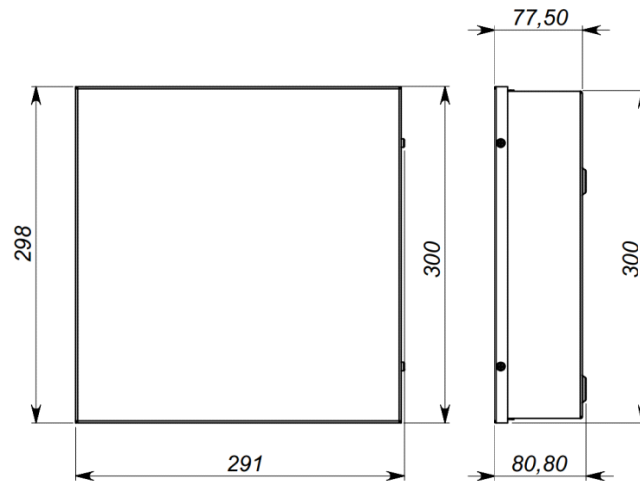
Рис 9. Габаритные размеры
