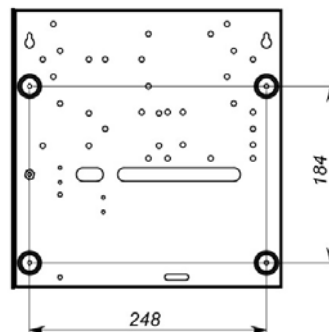
Рис 10. Разметка крепежных отверстий
