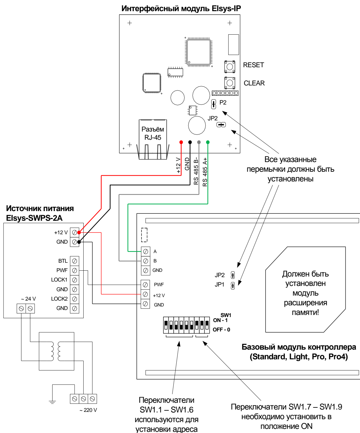
Рис. 4 – Схема подключения модуля Elsys-IP к контроллеру Elsys-MB
