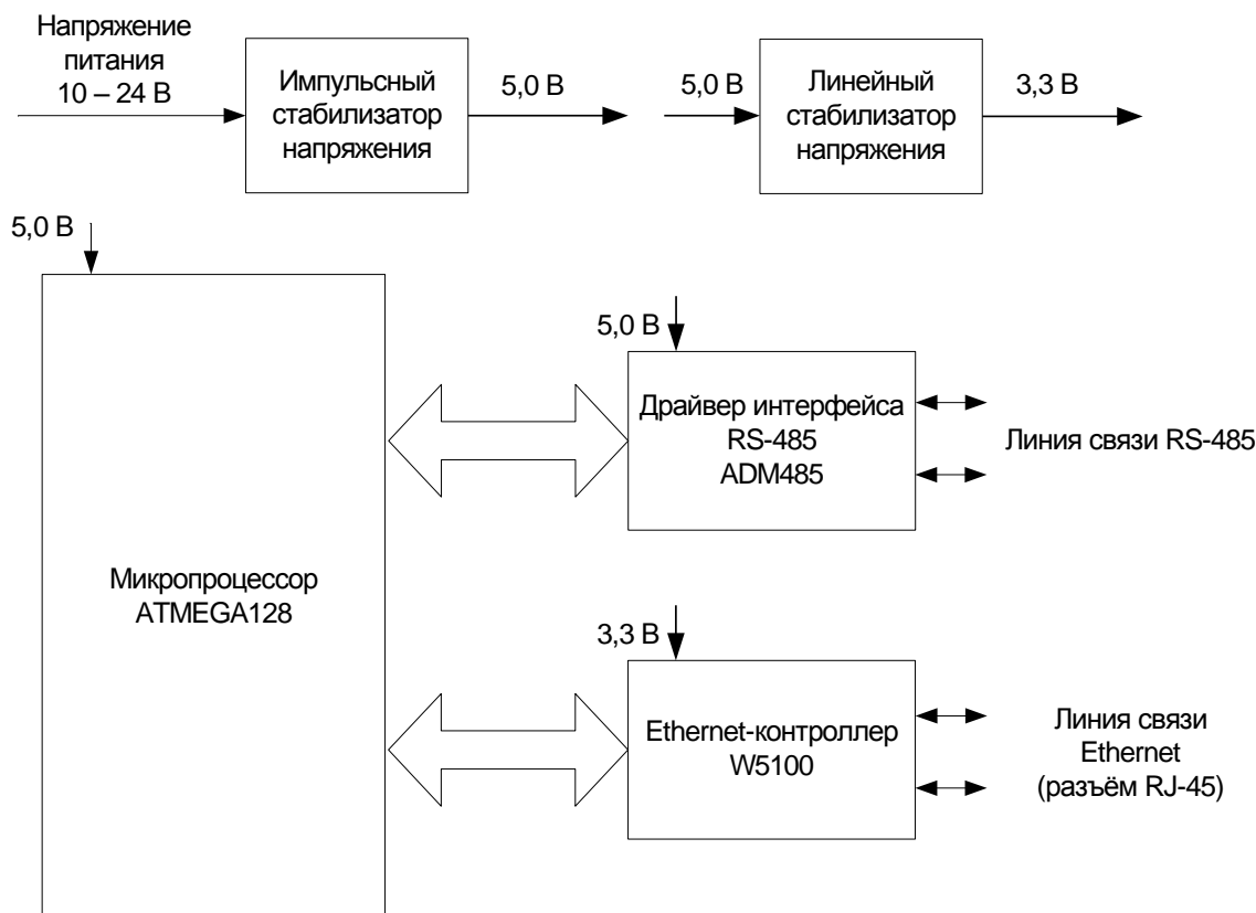
Рис. 1 – Функциональная схема модуля Elsys-IP
