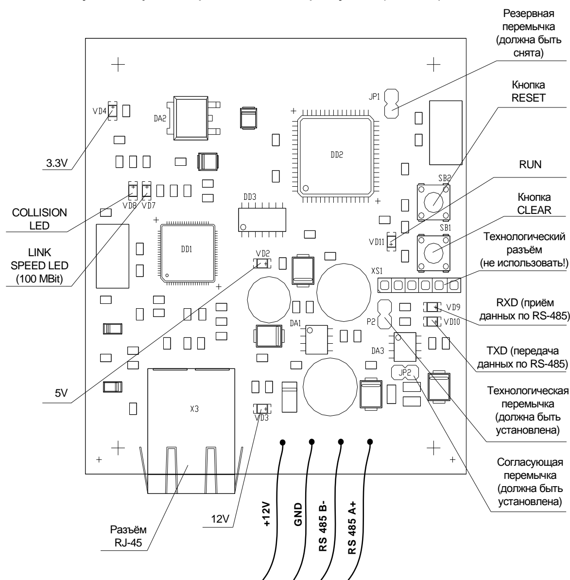
Рис. 3 – Схема расположения элементов модуля Elsys-IP
