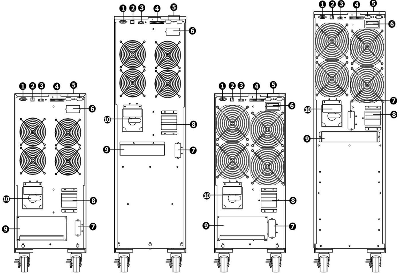
Рис.2-2 Внешний вид задней панели ИБП.
