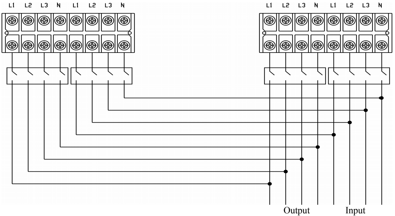
Рис.2-4-1 Подключение в параллельную систему ИБП XE 10 / 20 ( на примере двух ИБП).
