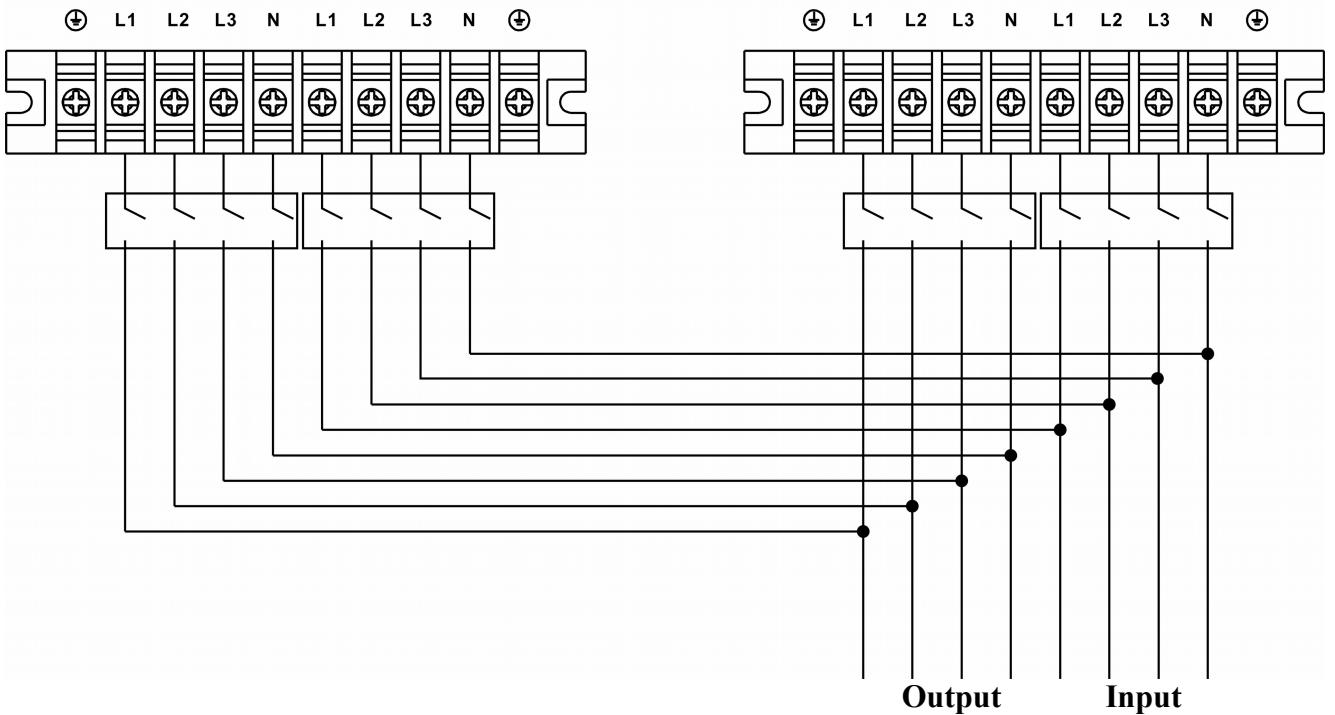
Рис.2-4-2 Подключение в параллельную систему ИБП XE 10WB/ 20WB (на примере двух ИБП).
