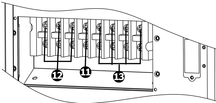
Рис.2-2 Внешний вид задней панели ИБП.
