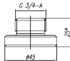
Рис. 8. Распылитель РСН-19-14,5-3/4
