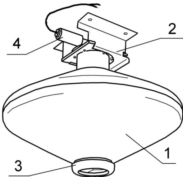
Рис. 1 – Конструкция МПП
