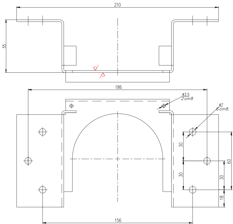
Рис. 3 - Крепёжная площадка МПП
