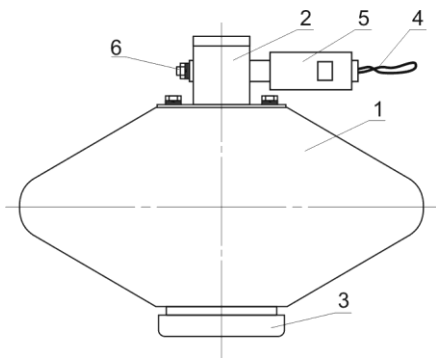
Рис. 1. Конструкция МПП «Гарант-5» во взрывозащищённом исполнении
