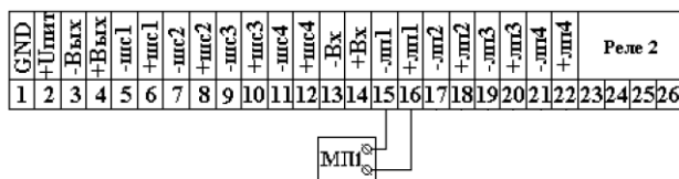
Рис. 11. Схема подключения МПП серии «Гарант» исп. 1 к прибору
