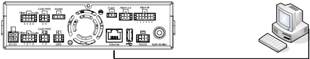
Рисунок 1-3 Прямое соединение ПК
