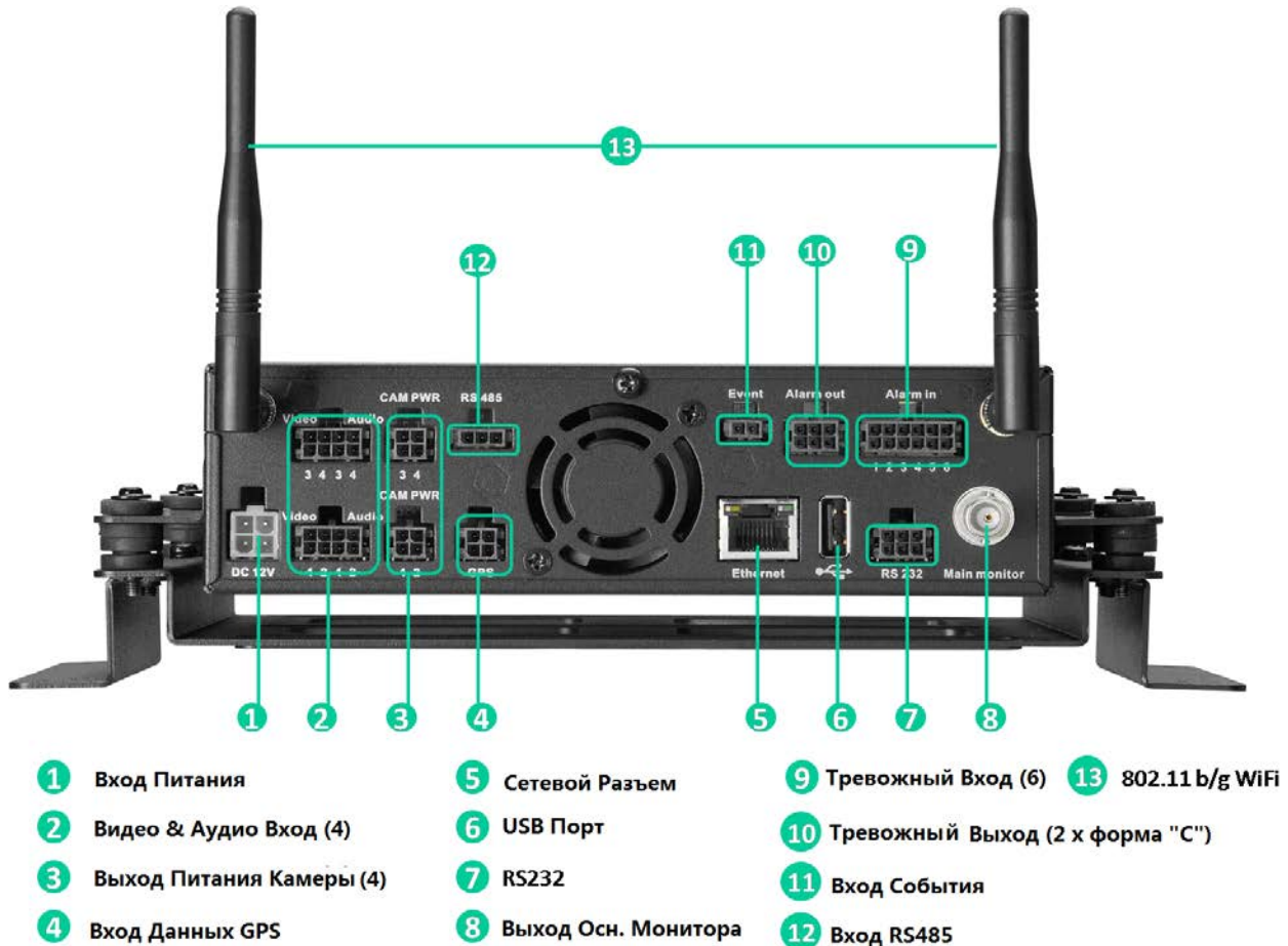
Рисунок 1-2 Задняя Панель
