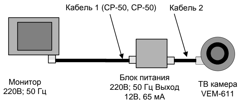
Рис.1. Схема включения камеры VEM-611.
