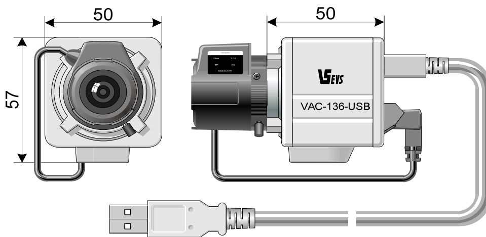
Рисунок 1 Внешний вид камеры VAC-136-USB, габаритные размеры.
