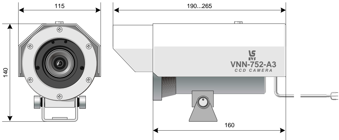
Рис.2. Камера VNN-752-A3 в металлическом корпусе
