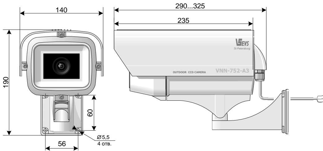
Рис.1. Камера VNN-752-A3 в пластмассовом корпусе.
