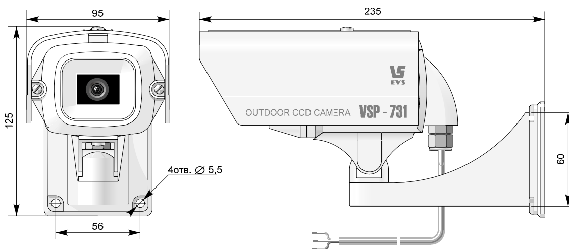
Рис.1. Камера VSP-731 .
