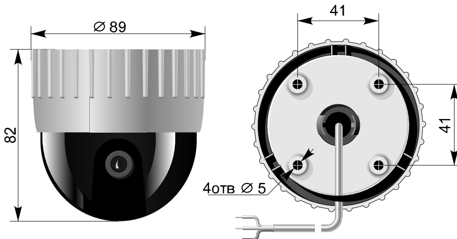
Рис.1. Камера VSS-531, вариант 1.
