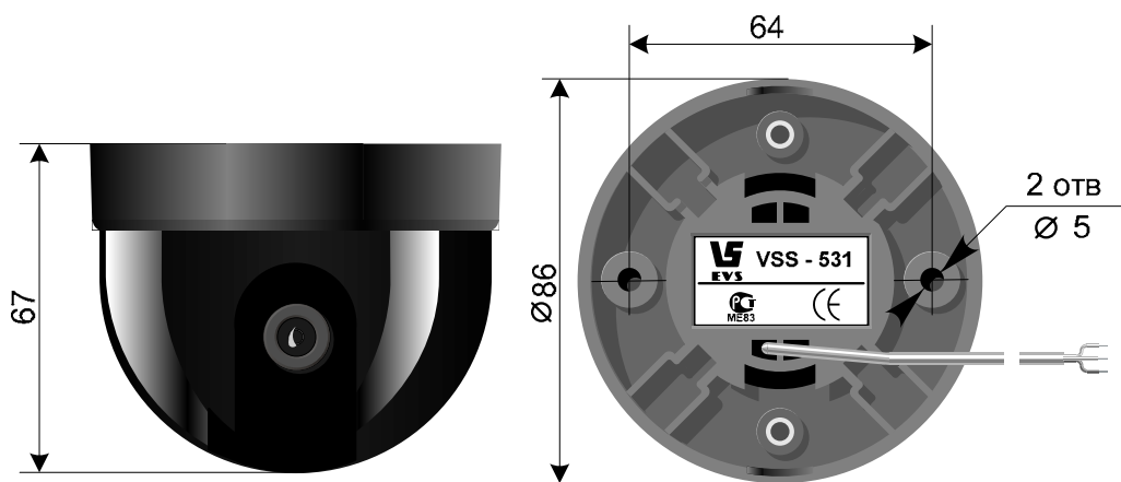
Рис.1. Камера VSS-531, вариант 1.
