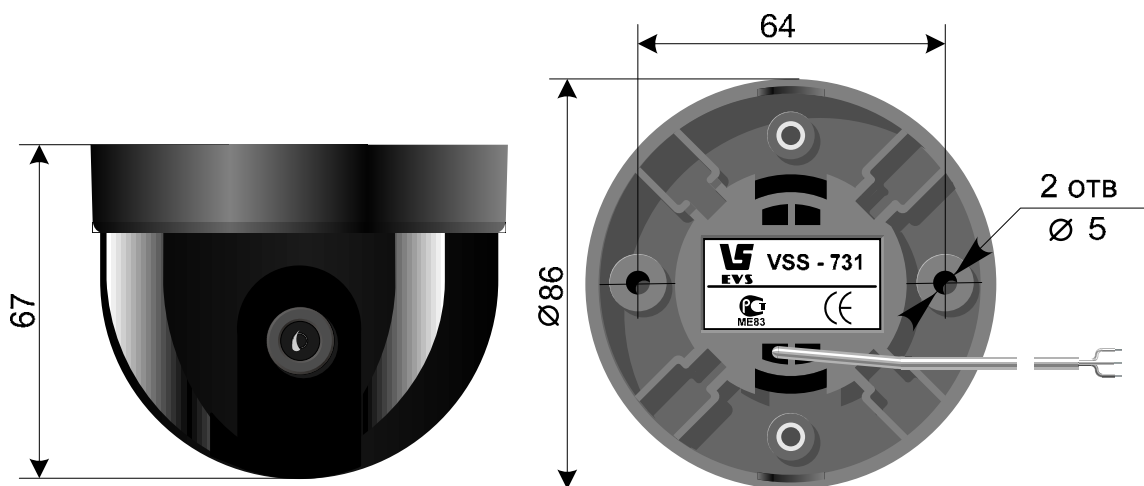
Рис.1. Камера VSS-731 вариант 1.
