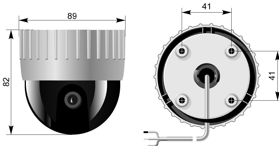
Рис.1. Камера VSS-731 вариант 1.
