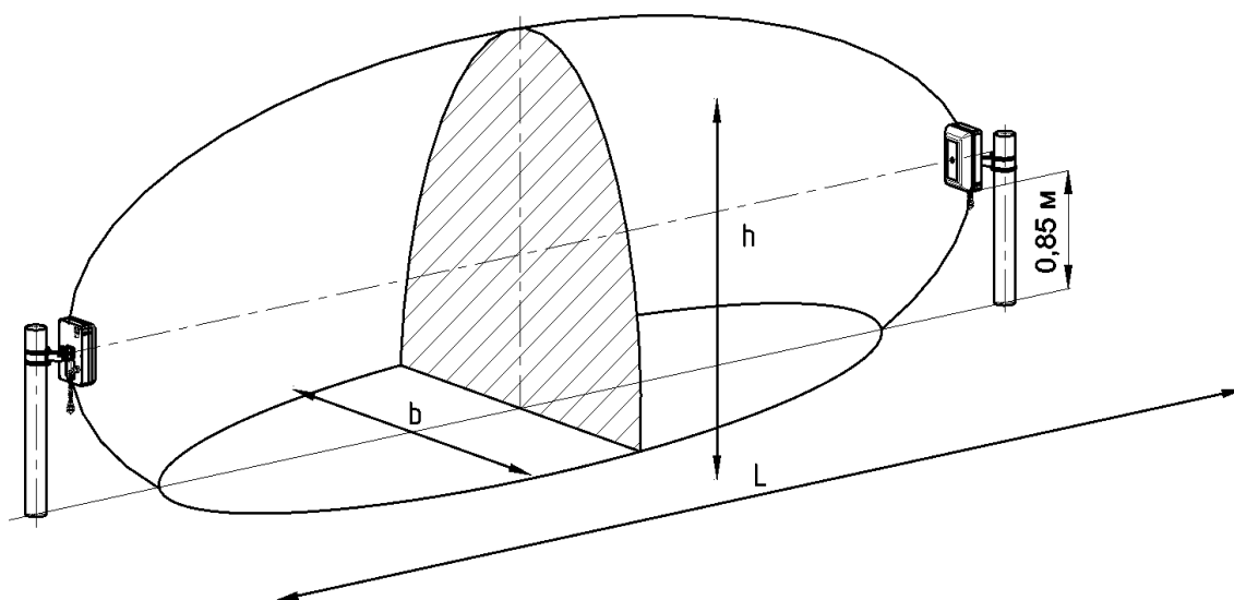
Рисунок 1.1 – Зона обнаружения извещателя
