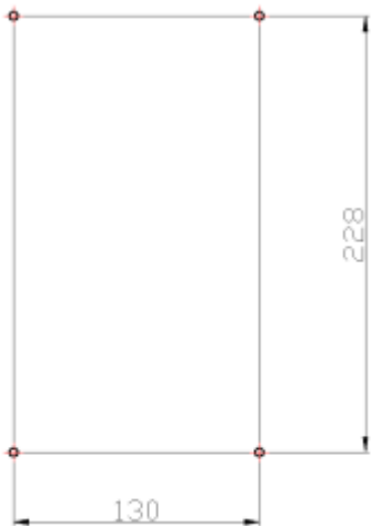
Рисунок 2.1. Разметка отверстий для крепления источника на плоской поверхности
