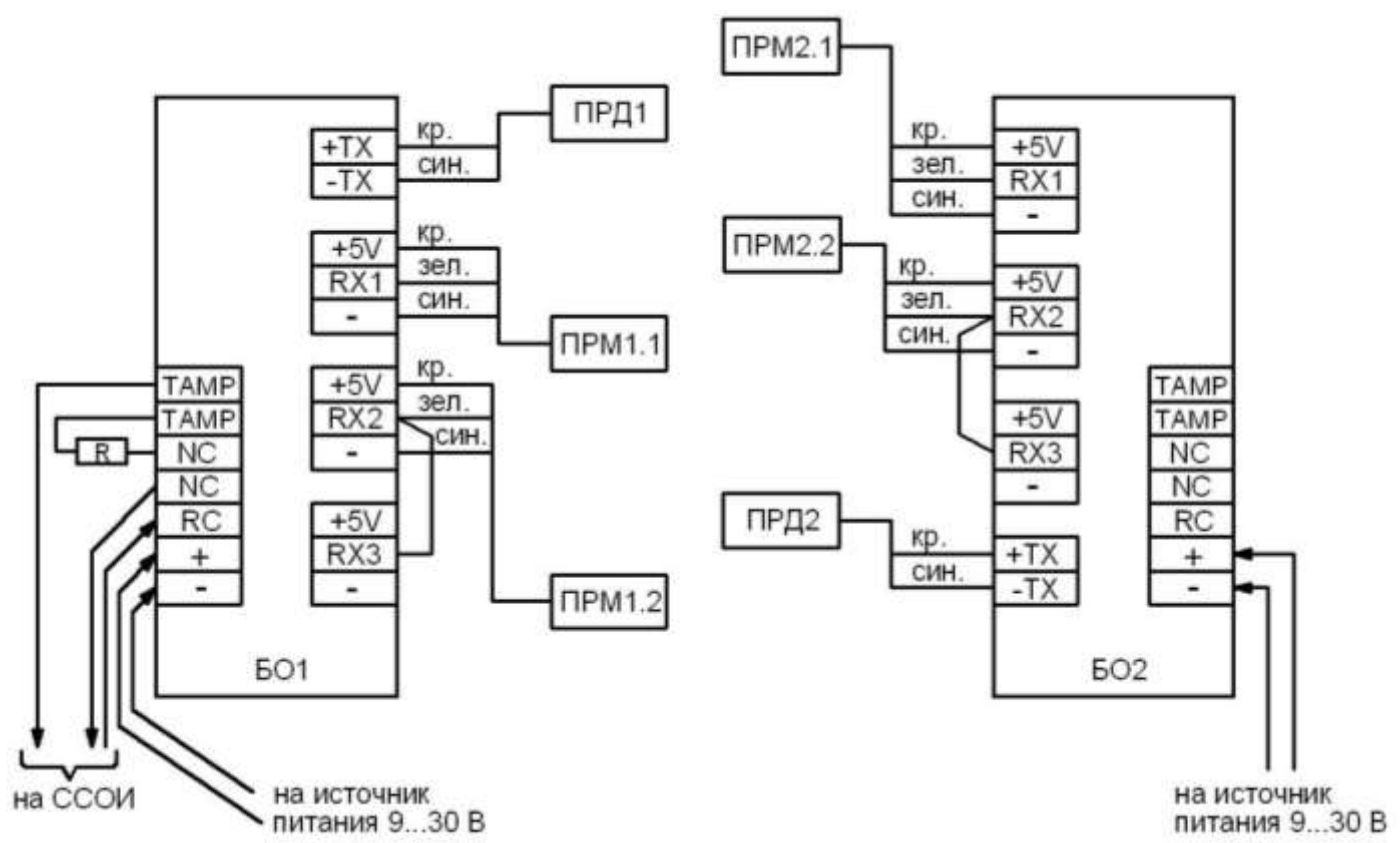
Рисунок 8.1 – Схема электромонтажа 4-лучевого извещателя.
