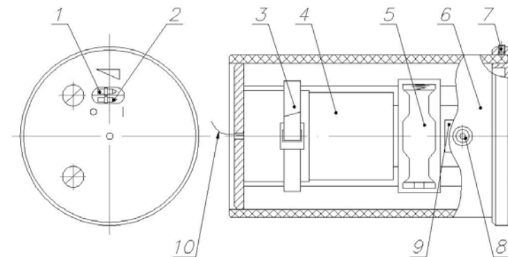
1— переключатель "Громкость"; 2— переключатель "Питание"; 3— стяжка; 4— катушка с микропроводом; 5— батарейный отсек с элементом питания; 6— корпус; 7— винт стопорный; 8— гнездо "ПЦН"; 9— колодка; 10— микропровод.
