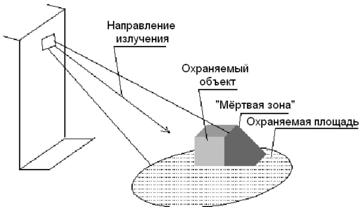
Рисунок 7.2 Расположение извещателя при установке на стене здания
