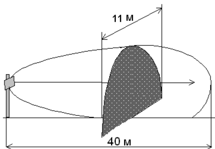
Рисунок 7.1 Зона обнаружения извещателя при установке на участке периметра
