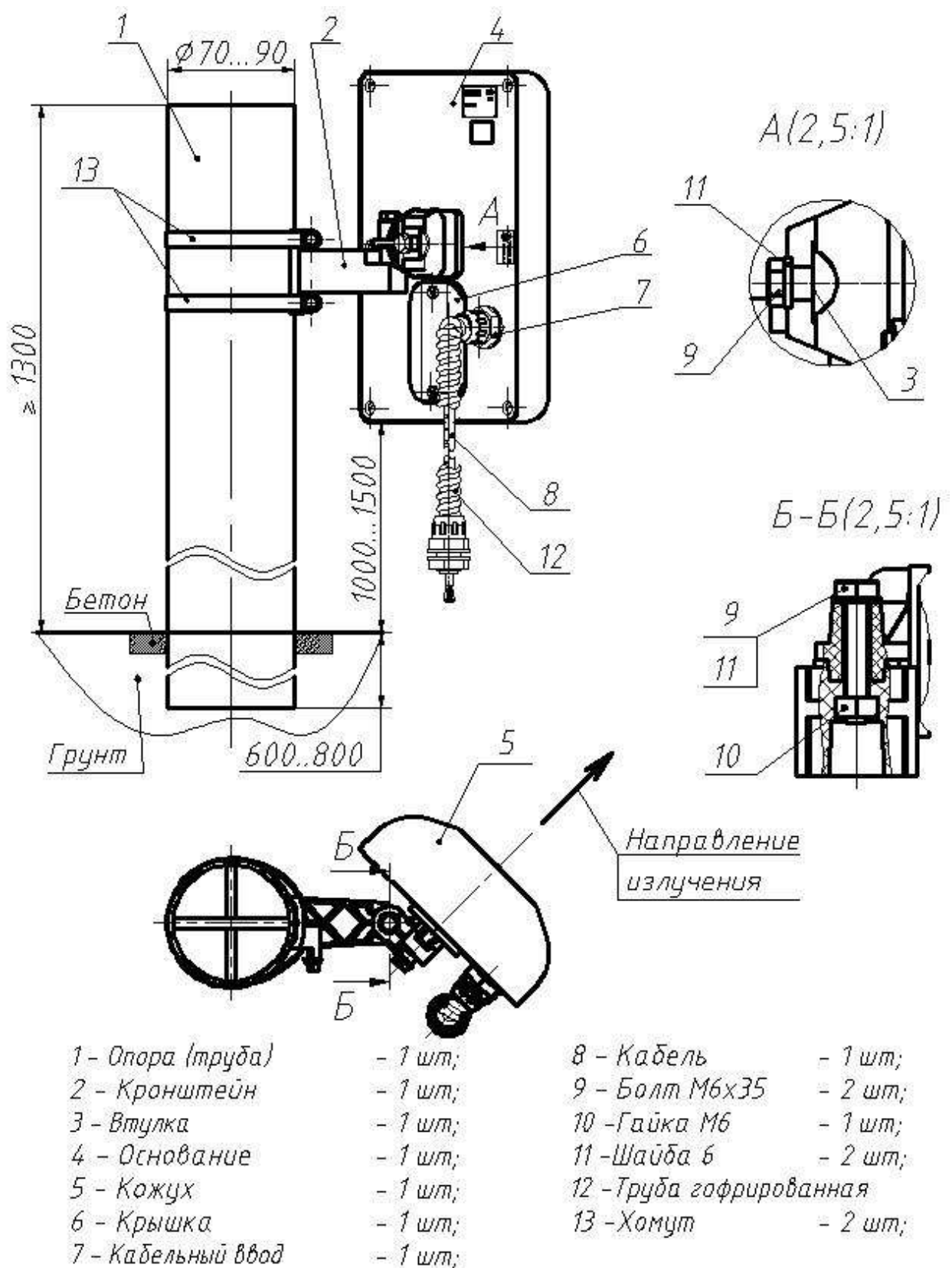
Рисунок 5.1 Установка извещателя на опоре
